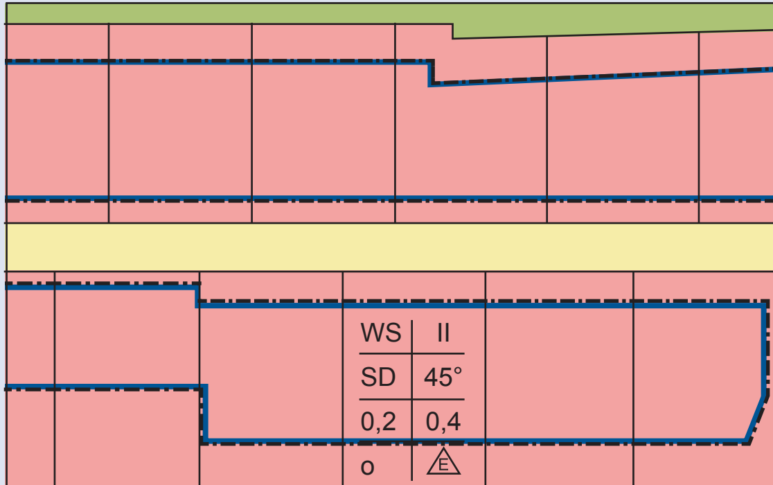
Bebauungsentwurf M 1:1000
