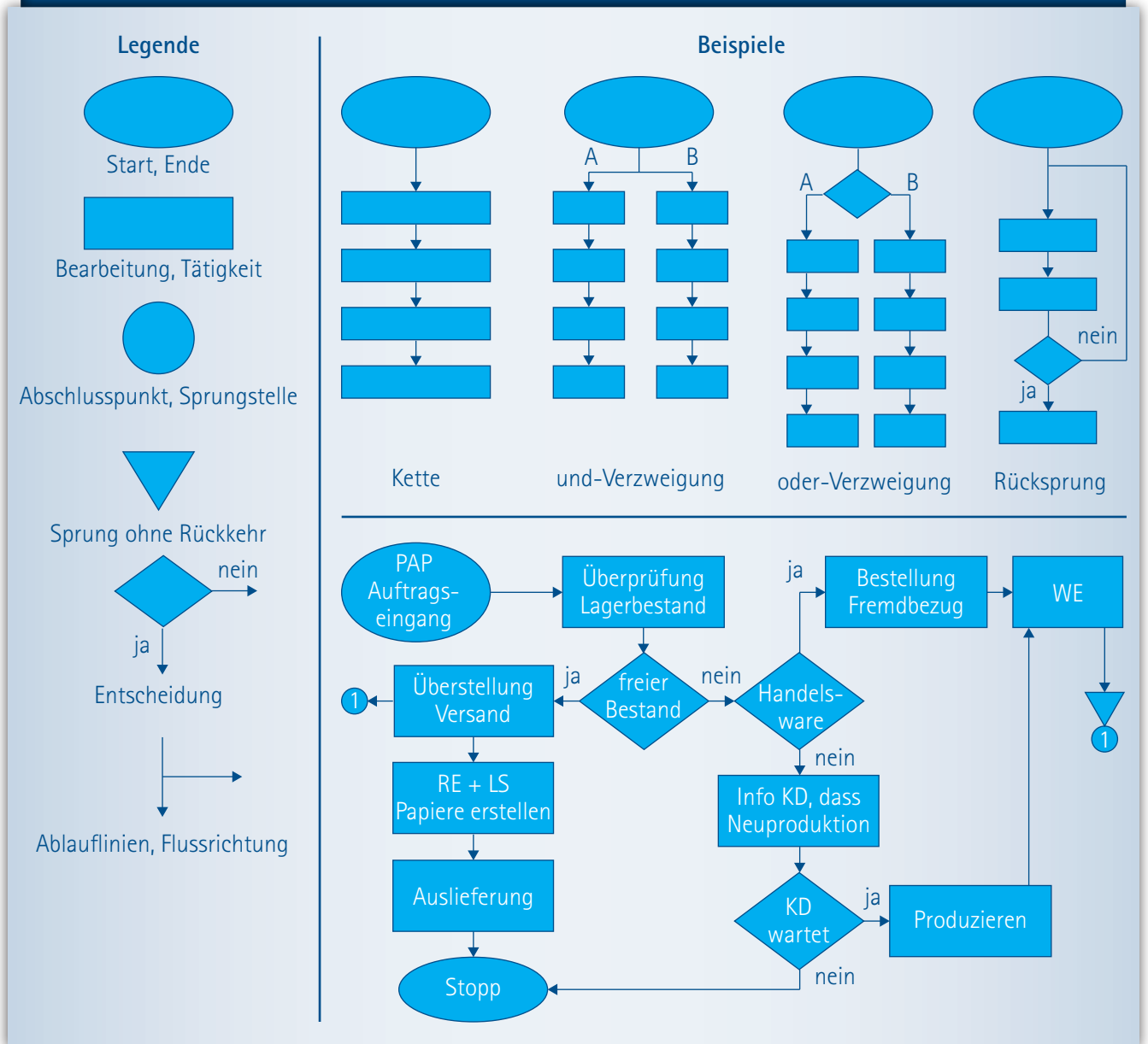
Abb. 0.4: Flussdiagramme (Symbole nach DIN 66001)
