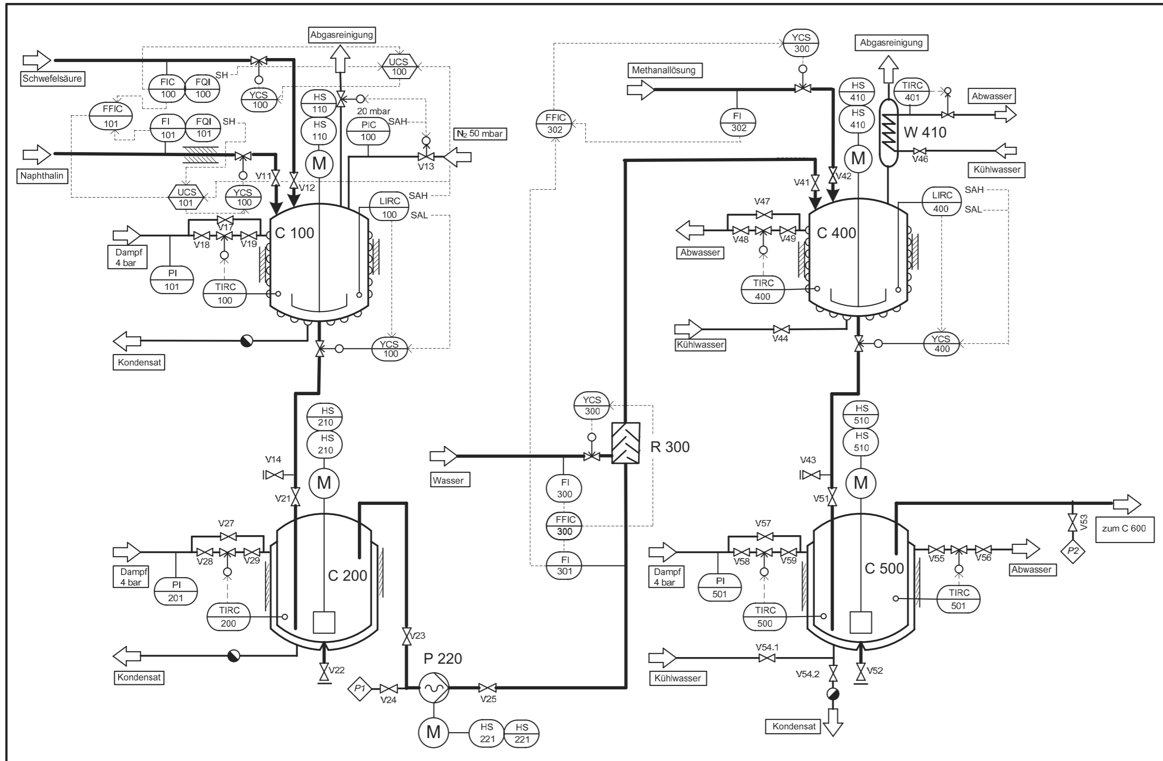
Kesselkaskade zur Herstellung von Polynaphthalinsulfonsäuren
