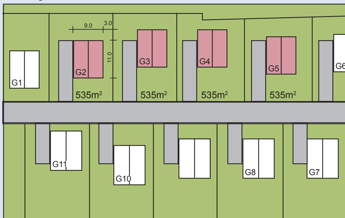
Bebauungsentwurf M 1:1000
