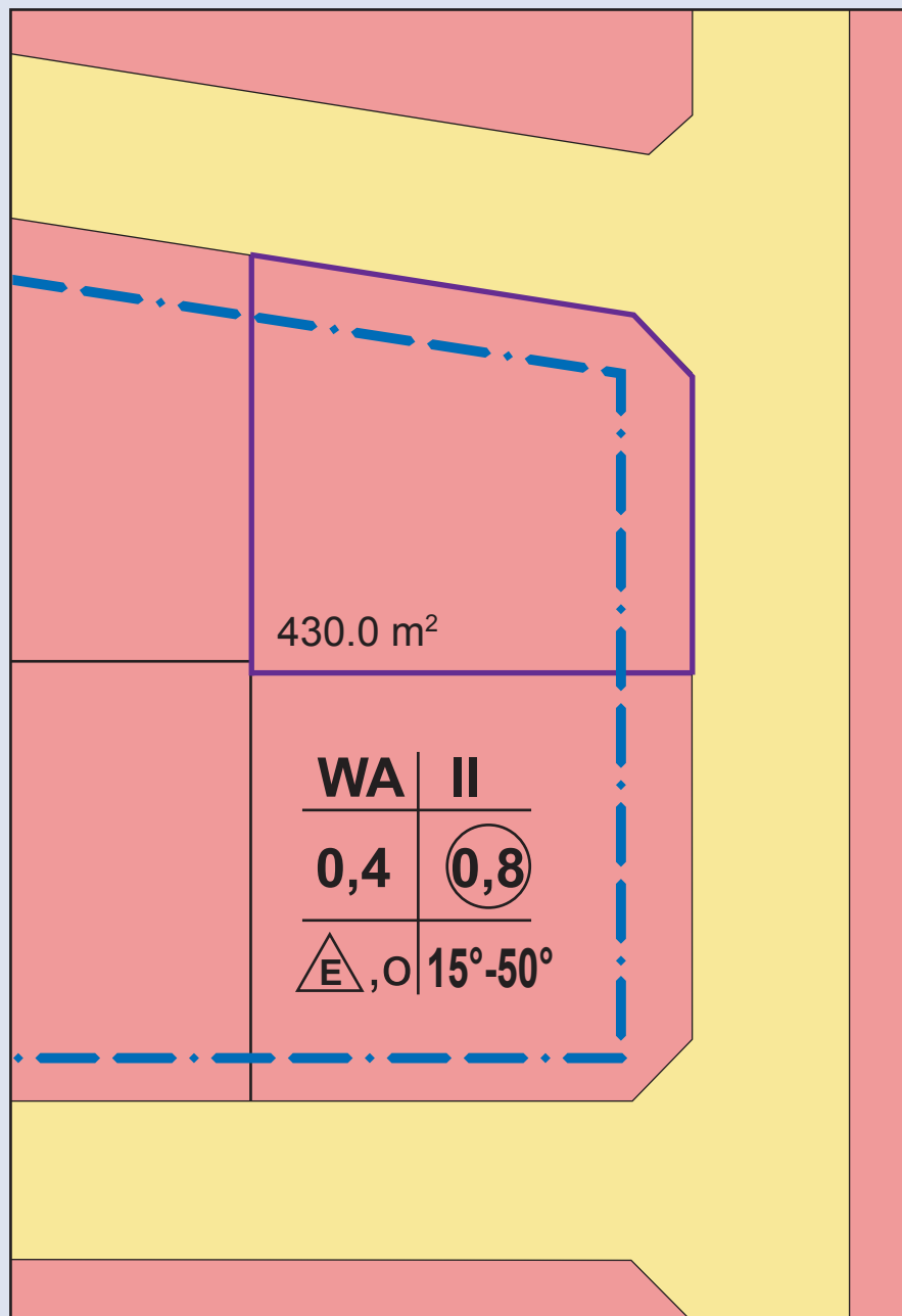
B-Plan Auszug
